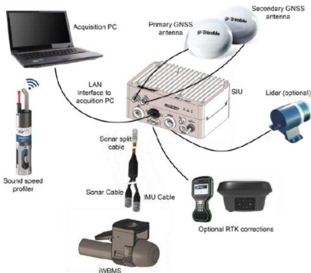
Figura 9 Componentes ecosonda Norbit
