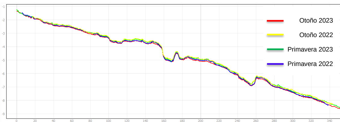
Figura 11 Batimetrías perfil 1
