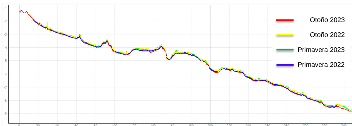
Figura 12 Batimetrías perfil 2
