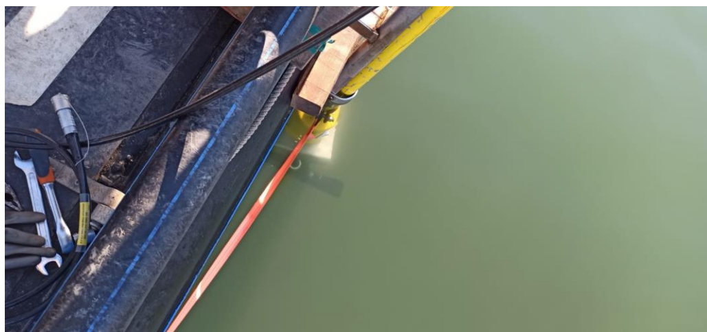
Figura 5 Montaje de la MBES en la embarcación.
