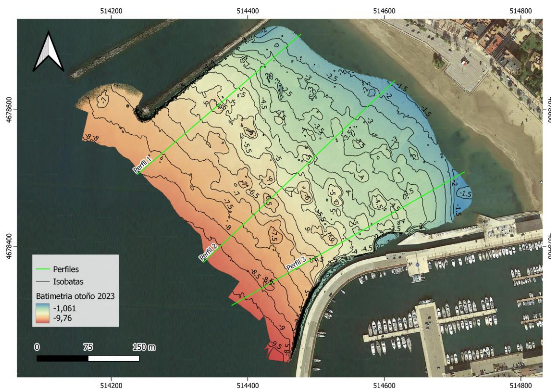
Figura 10 Batimetría y perfiles
